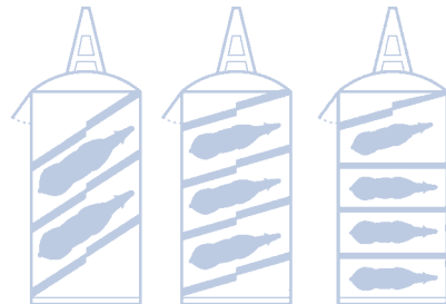
Anordnungsbeispiele für Trennwände im HB510XL
